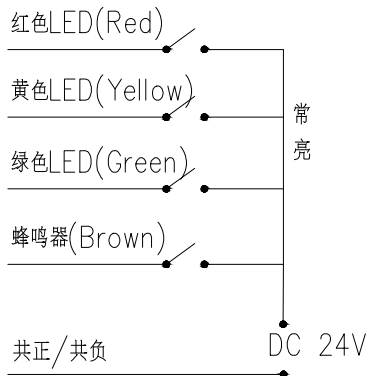
接线图
