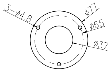
安装尺寸
