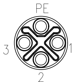
S扣母插孔图
