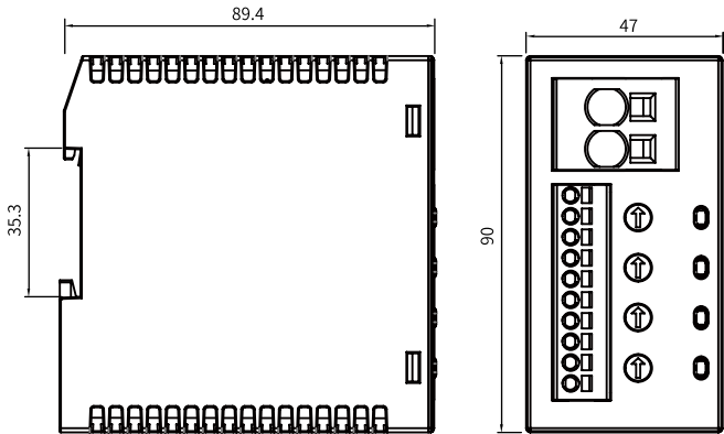
PRB410/PRB411 Dimensions
